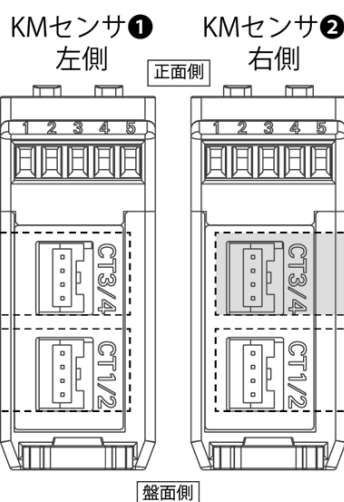
KMセンサ 本体下面
