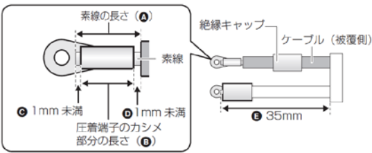
図7. 圧着端子とケーブルの加工
