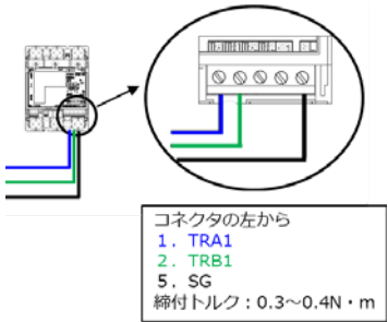
図5. Modbus通信ケーブル配線（S2MS、S3MS）
