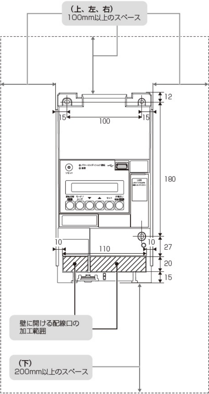
取り付け寸法図 (単位: mm)
