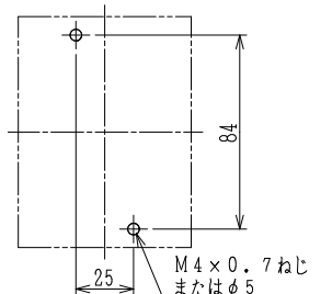
【単位：mm】
