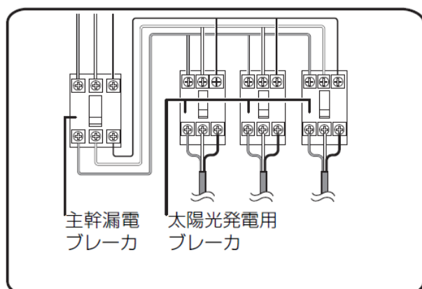
集電箱の例
