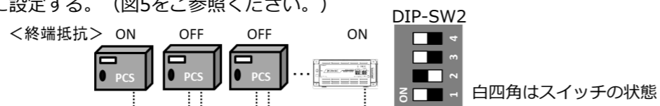
図5. 終端抵抗の設定 (パターンAの場合)
