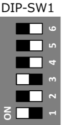
図10. DIP-SW1
