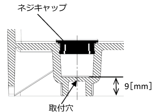
図3. 取付穴加工図
