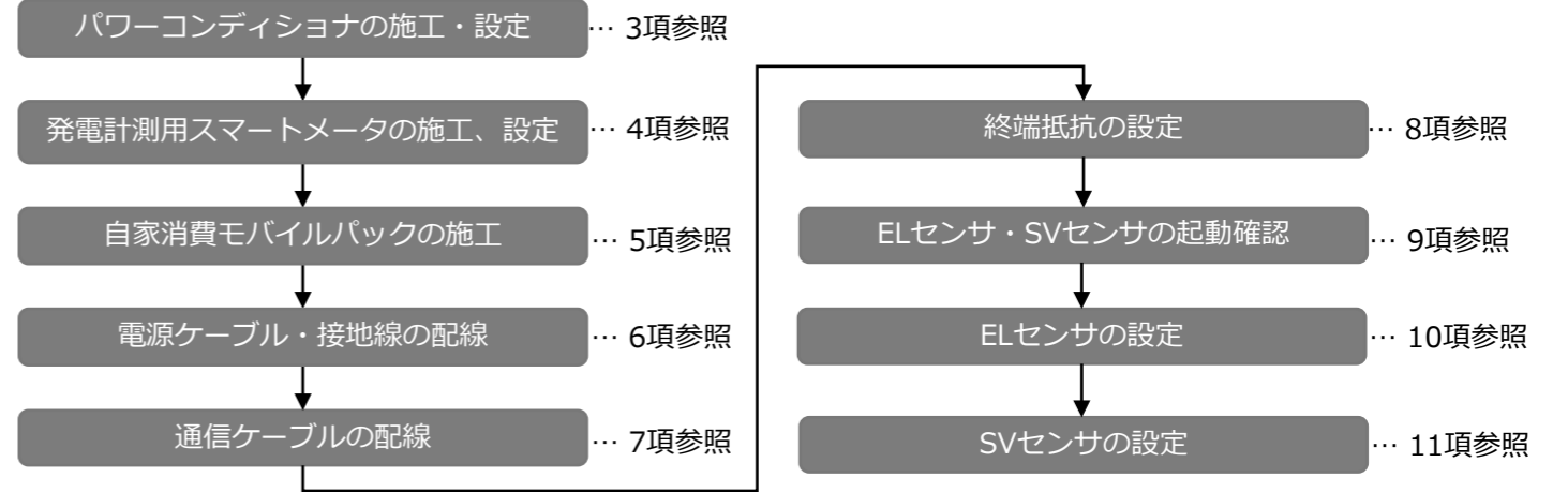
図1. 自家消費モバイルパック施工の流れ
