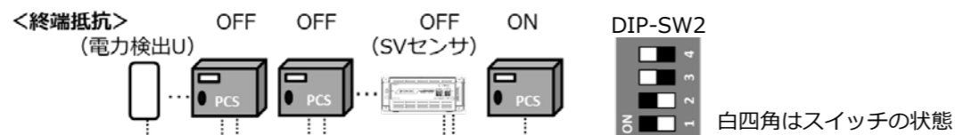
図4. 終端抵抗の設定 (パターンBの場合)
