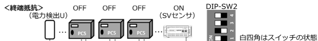
図3. 終端抵抗の設定 (パターンAの場合)
