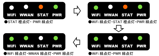
図7 リセット実施後のLED点灯パターン(正常時)
