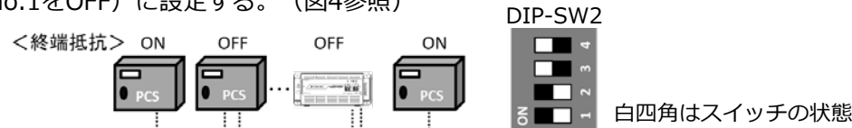
図4. 終端抵抗の設定 (パターンBの場合)
