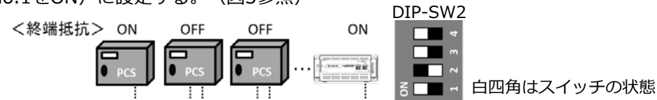
図3. 終端抵抗の設定 (パターンAの場合)
