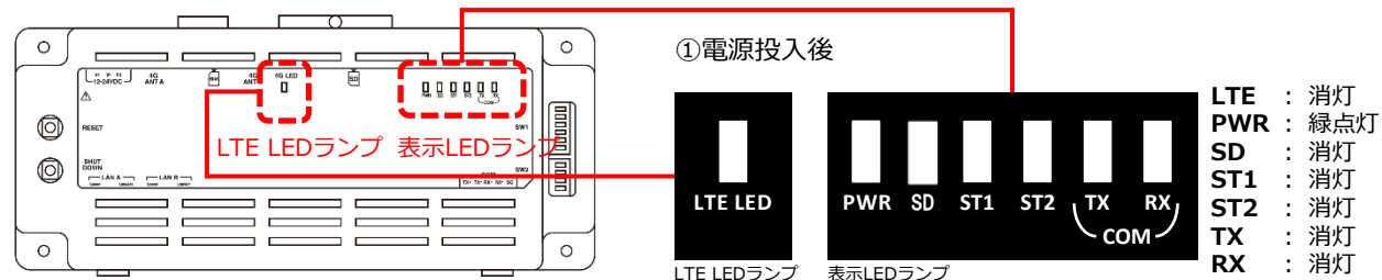
図6. SVセンサ ランプ位置
